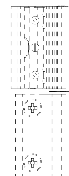
00136 FLUSH BASE HINGES
