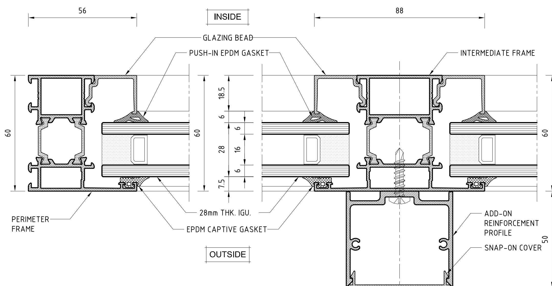
JAMB DETAIL
